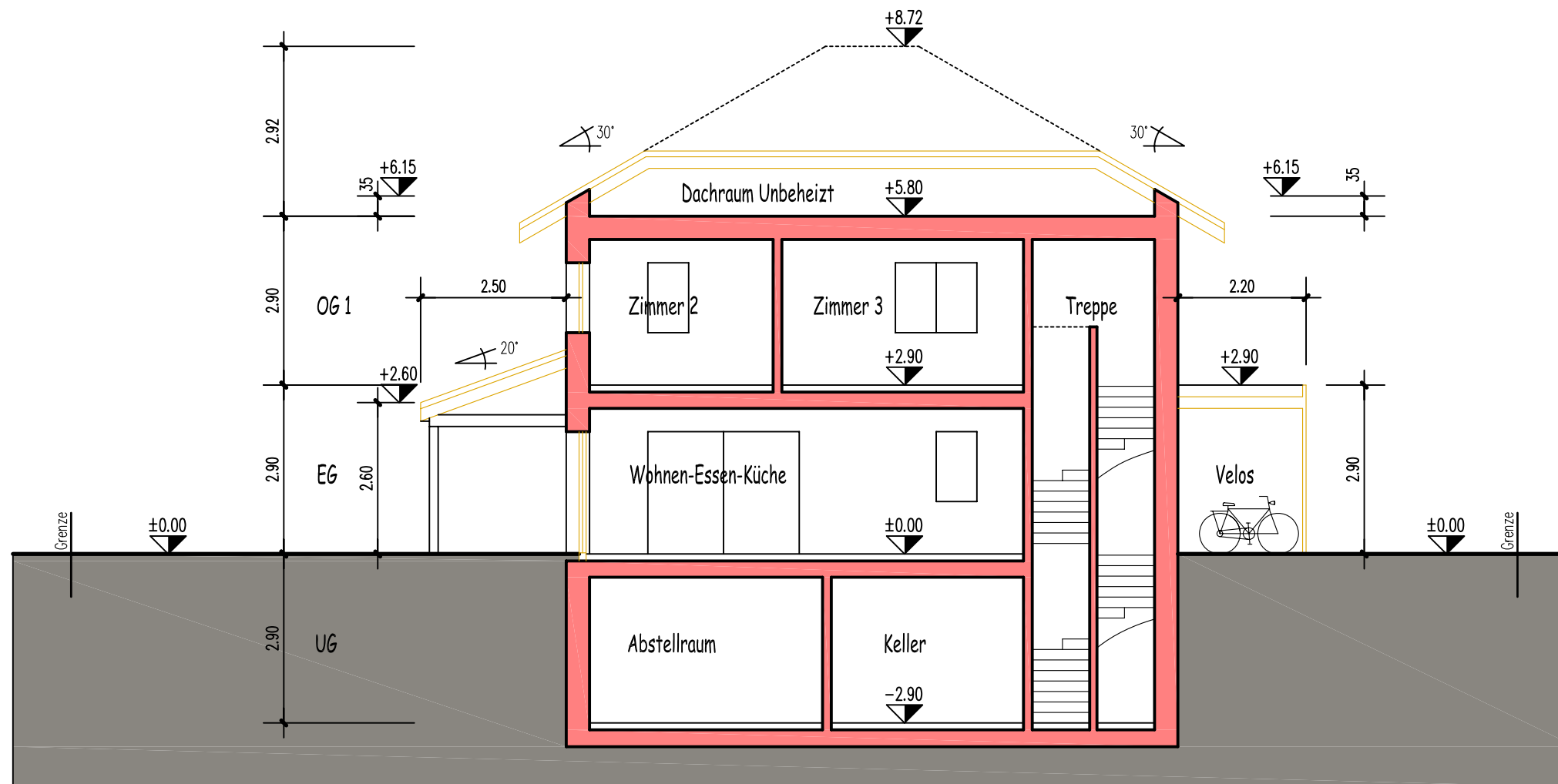
Schnitt B-B
