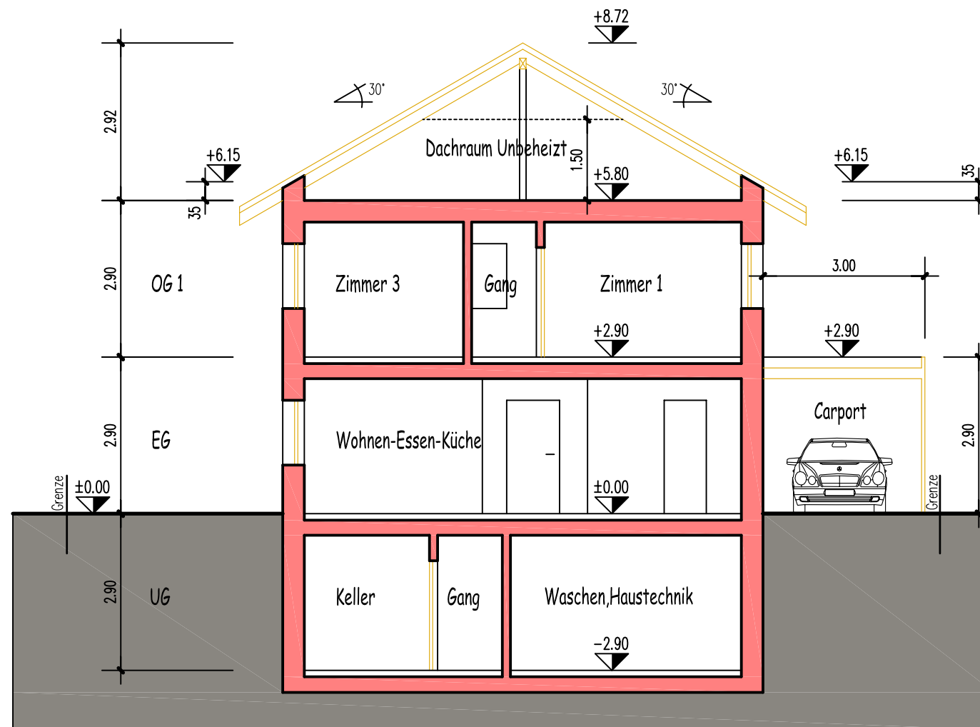
Schnitt A-A
