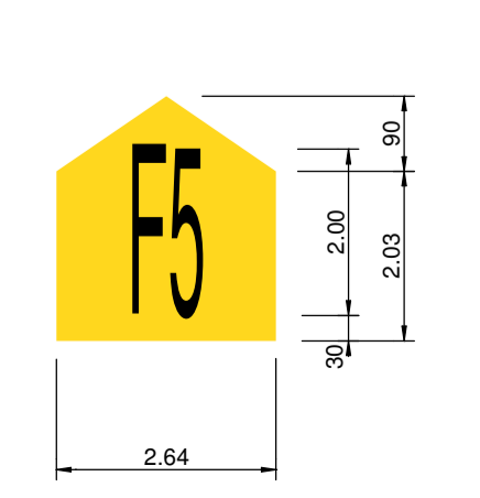
Detail ⑤ : Standplatz-Bezeichnung 1:100
