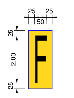
Detail ④ : Taxilane 1:100
